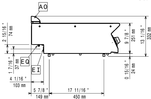
侧视
